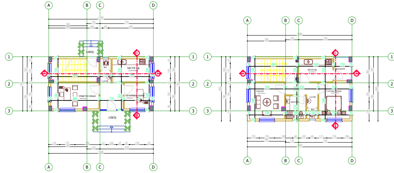
BAKICI EVİ 1.KAT PLANI
